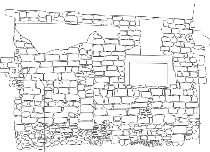
ALÇAT FRONTAL PARAMENT PART POSTERIOR CAL MANEL INT. ARQUEOLÒGICA CAL METGE SOLÉ I CAL MORATÓ (2010)
